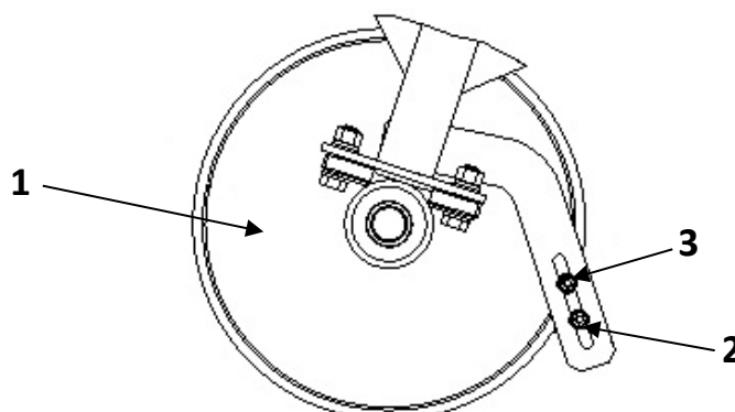
Rys. 9. Regulacja ustawienia skrobaka wału ugniatającego.
