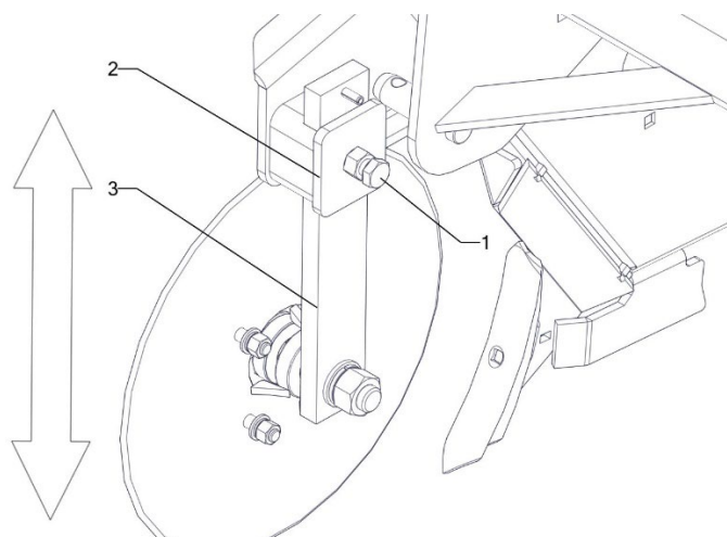
Rys. 8. Regulacja wysokości krojów.
