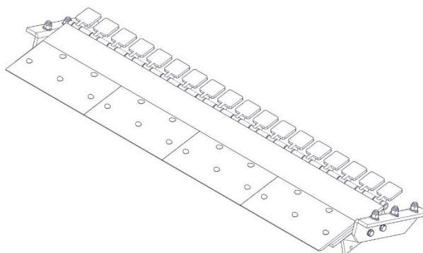
Rys. 6. Lemiesz listwowy.
