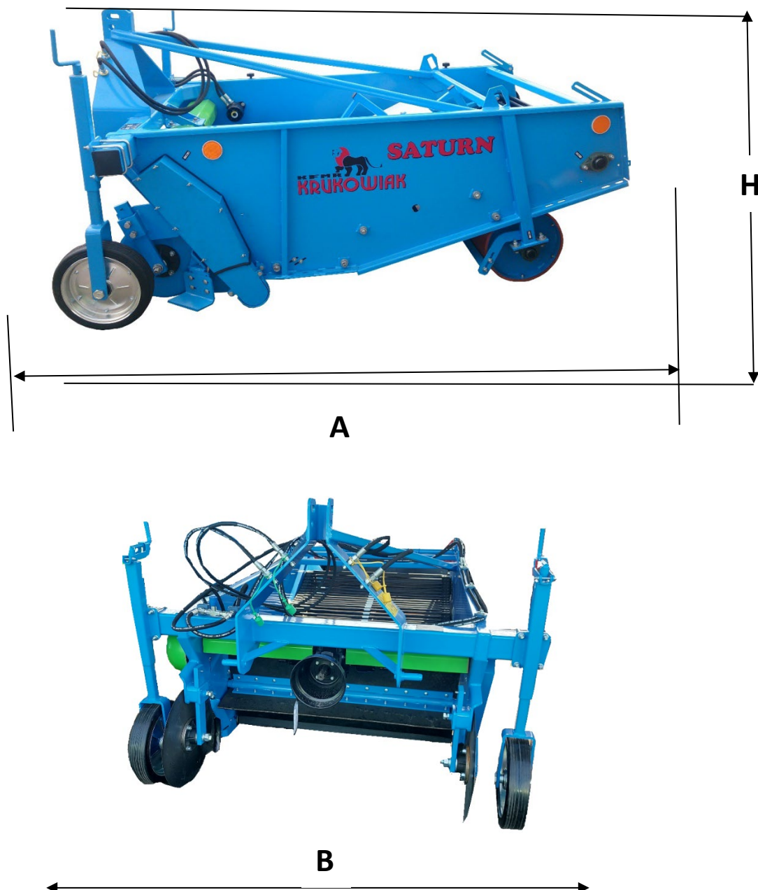
Rys. 7. Gabaryty w pozycji transportowej
