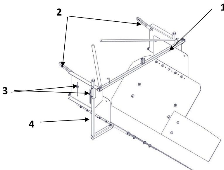
Rys. 10. Regulacja ustawienia formownicy (standard)
