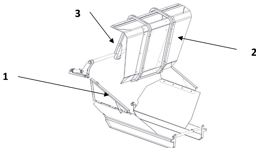
Rys. 12. Formownica zamykana hydraulicznie (opcja)
