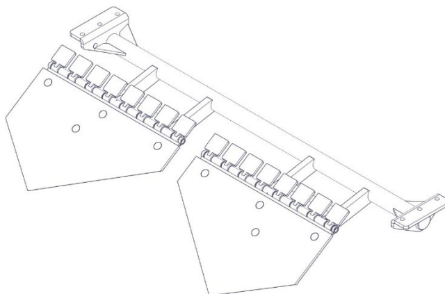
Rys.4. Lemiesz 2-częściowy
