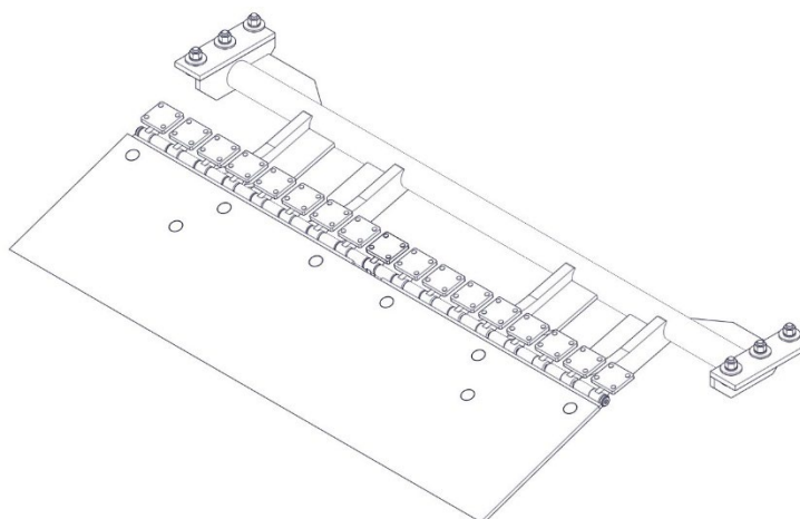
Rys. 6. Lemiesz listwowy do cebuli.
